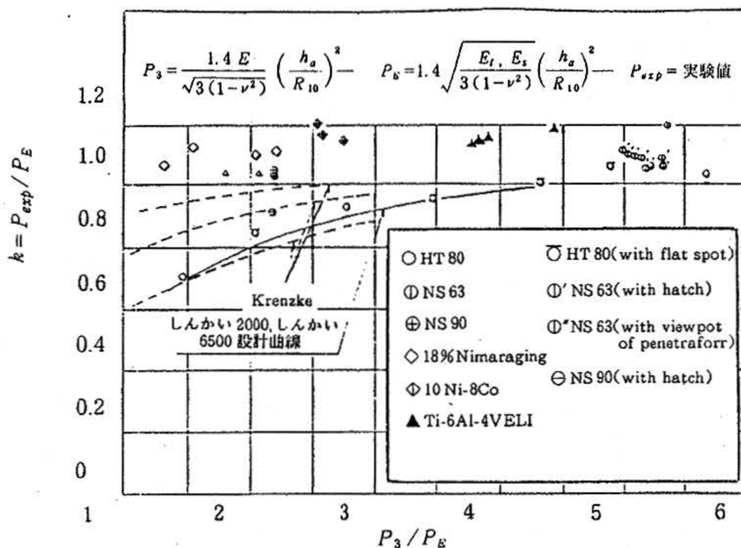
図2 球殻の圧壊強度比較
