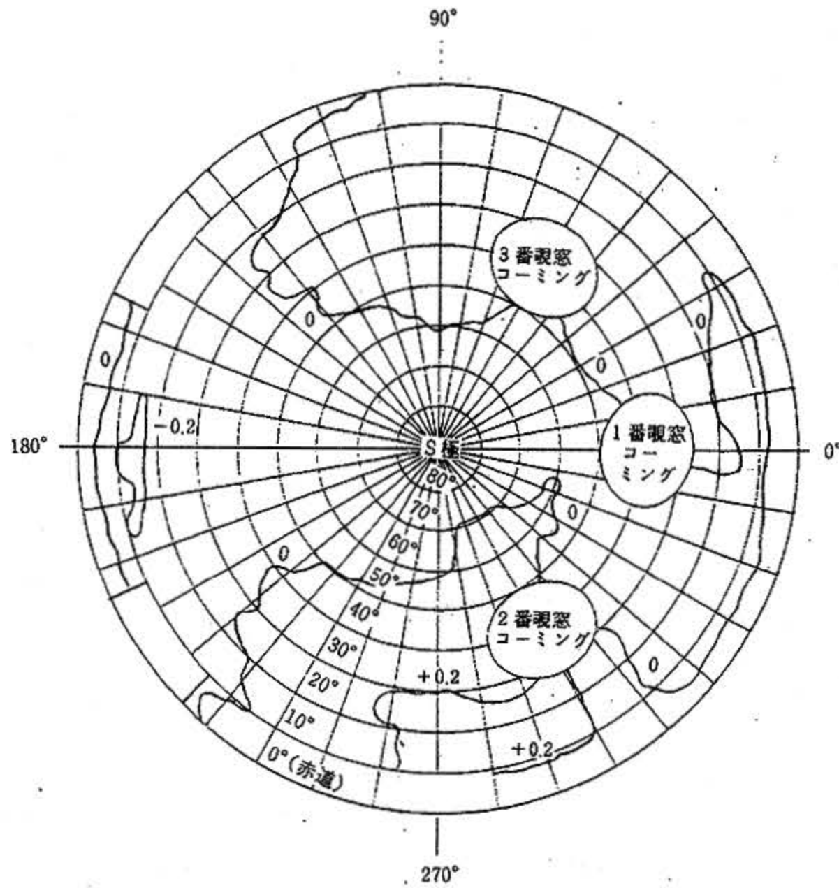
図8 耐圧殻S半球の真球からの半径偏差分布 Fig.8 Sphericity Deviation (Radius) Distribution of S-Hemisphere
