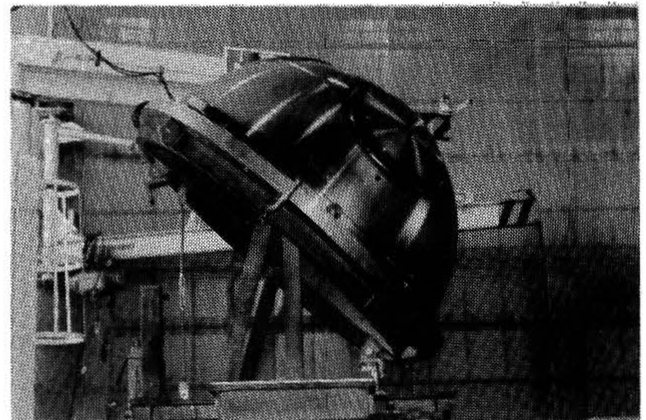
写真2 貫通金物嵌め込み溶接状況
