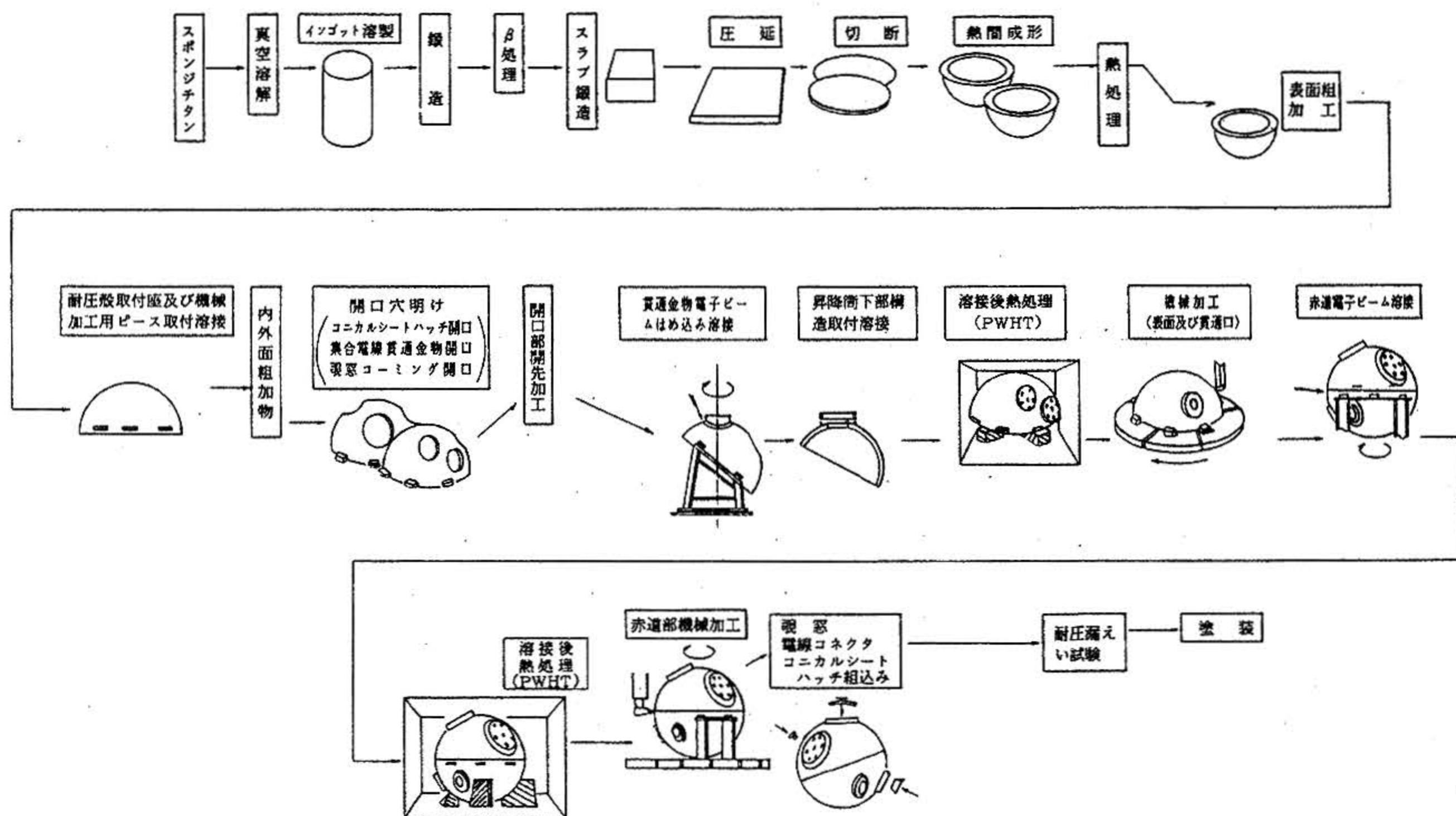
図6 耐圧殻製造手順
