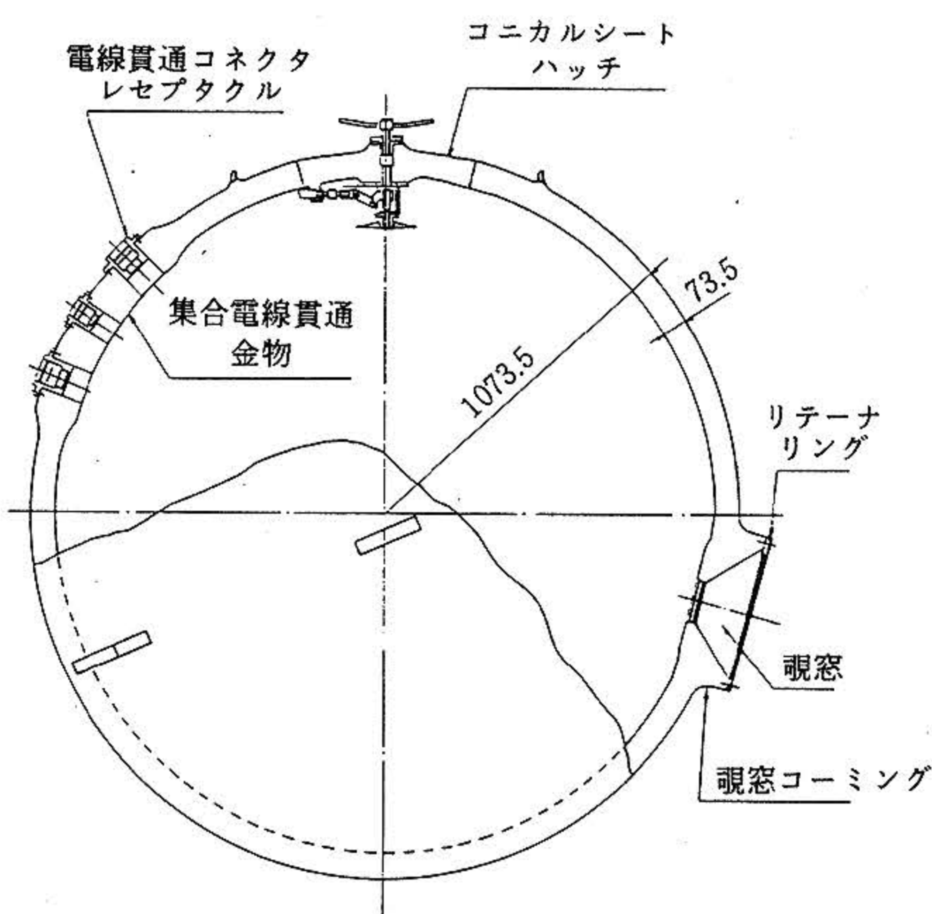
図1 耐圧殻概略形状図
