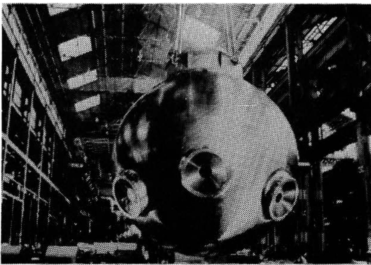
写真5 耐圧殻完成状態外観
