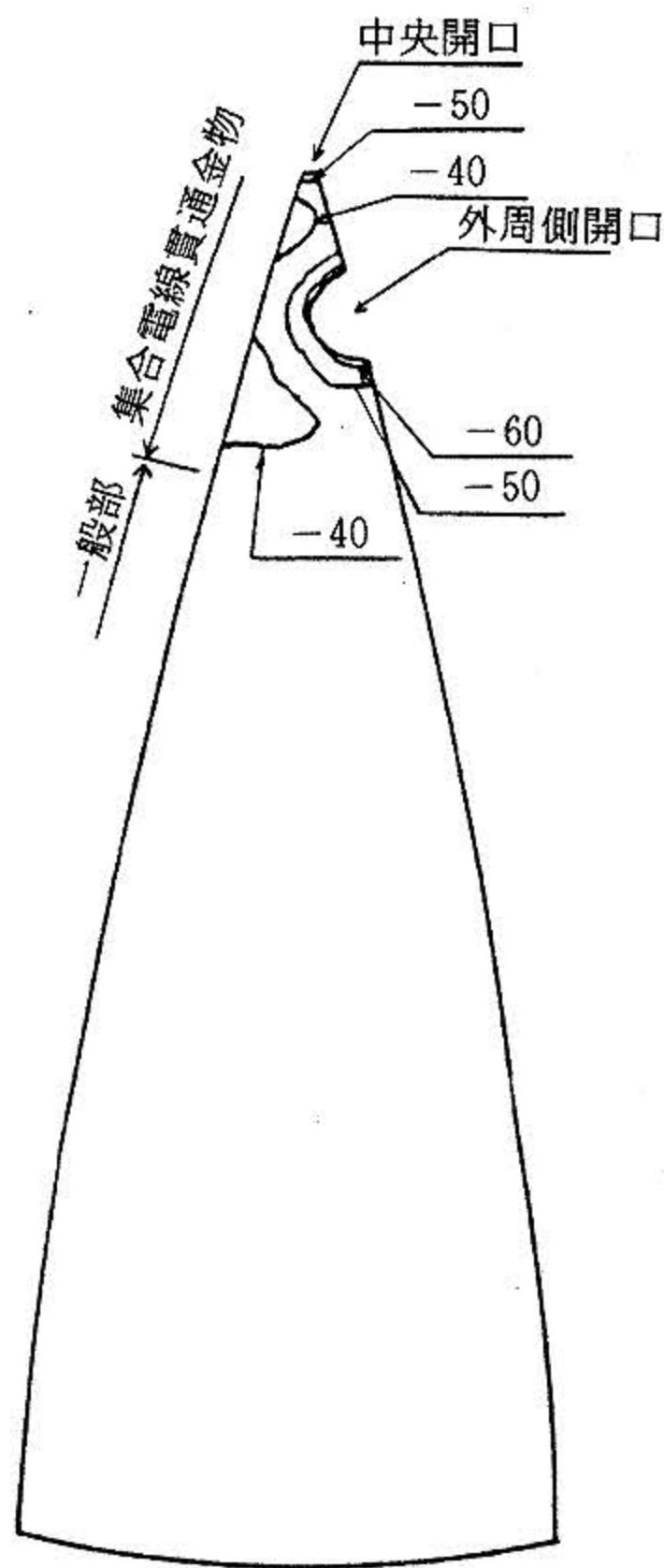
図5 最大主応力等高線図 (外圧 680 kgf/cm 2 ) Fig.5 Contour of Maximum Main Stress (680 kgf/cm 2 )
