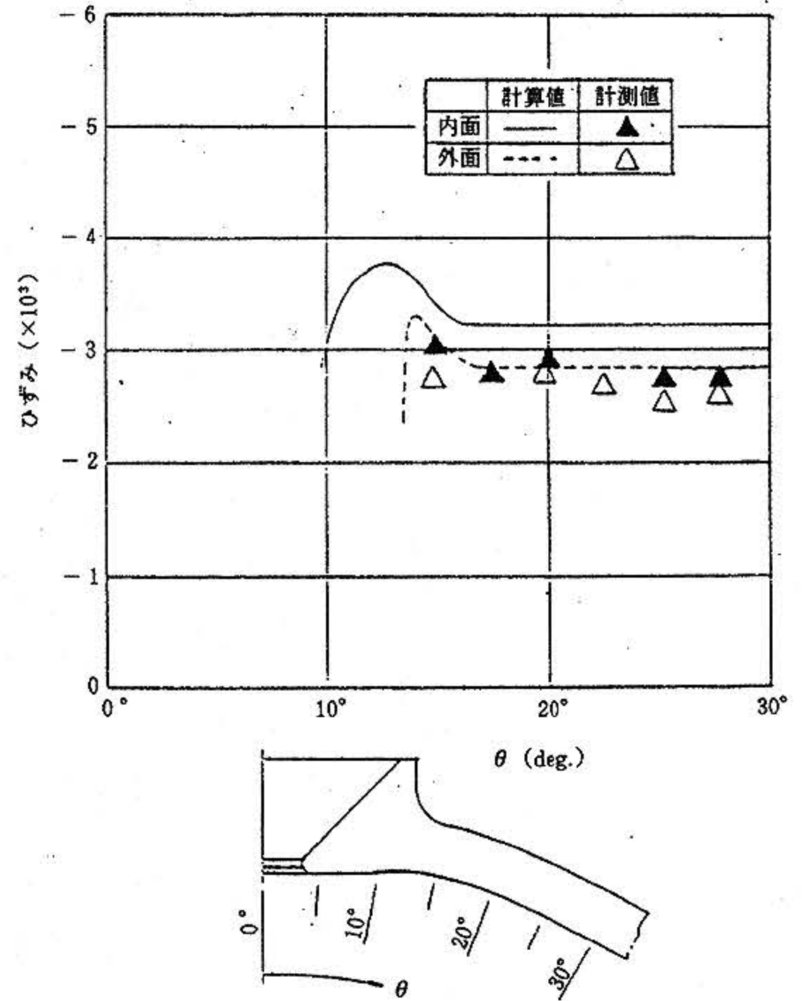
図13 視窓コーミング近傍経線方向ひずみ分布 (外圧 680 kgf/cm²) Fig.13 Longitudinal Strain Distribution Around Viewport Coaming
