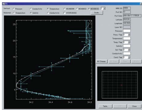
図9 フロートデータ品質管理プログラムの表示例:フロートデータと歴史的データ(WOA98)との比較画面 Fig. 9 Sample screen shot of the "Float data quality control program." Comparison graph of Float data and historical data (WOA98).
