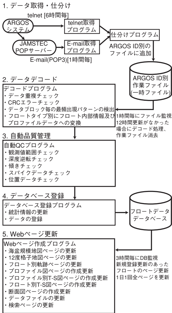
図3 自動データ処理のフローチャート Fig. 3 Flowchart of automatic float data processing.
