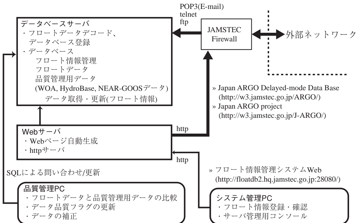
図1 フロートデータ処理システムの概要
