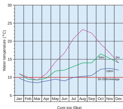
図4 回帰式によって求められた完新世0kaと最終氷期18kaの水深別年間水温
