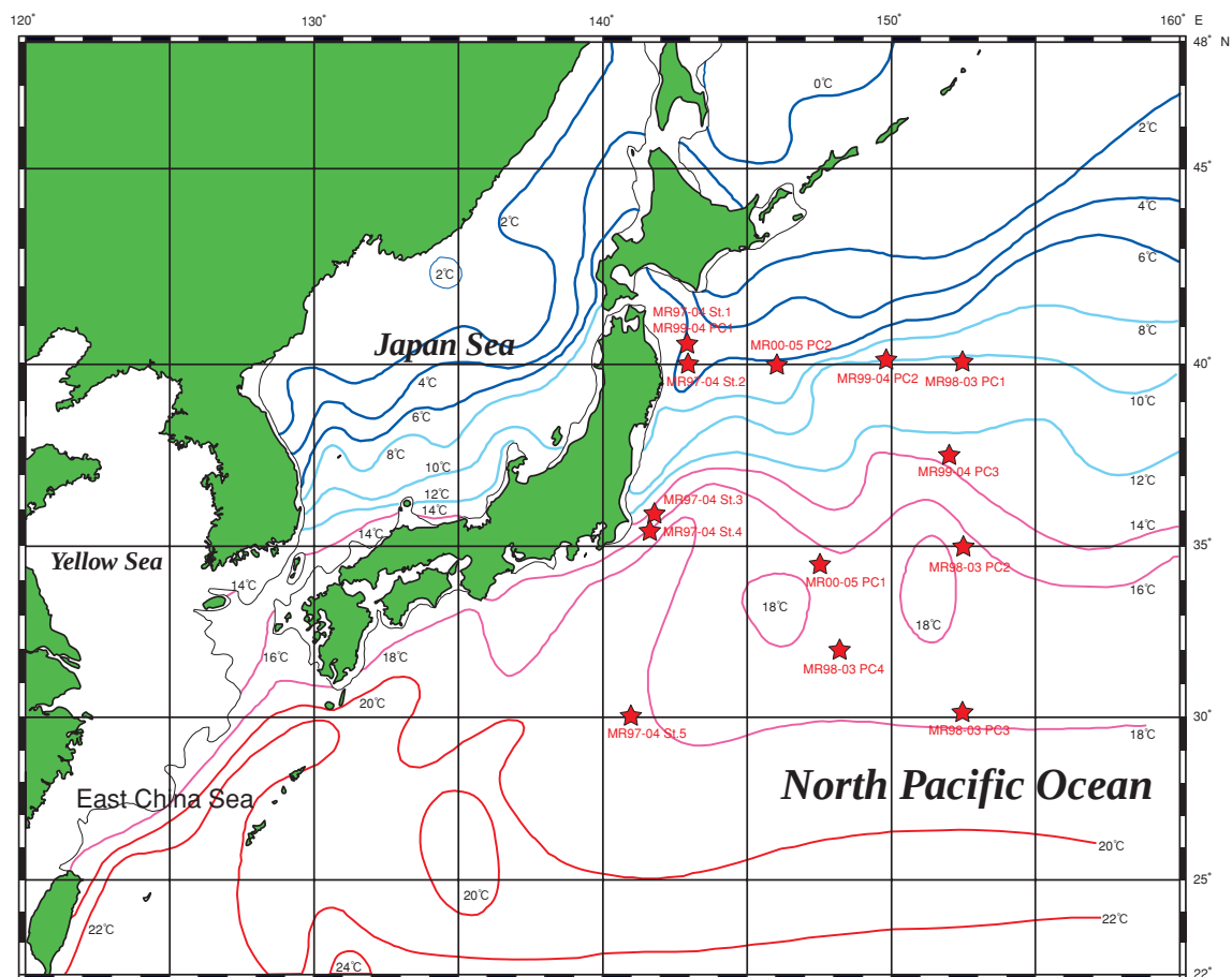
図2 みらいのピストンコア採泥点と春季100mの等温線(海洋環境図:1978改編)
