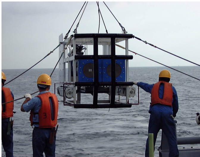
Deep Tow Sonar ディープ・トウ ソナー
