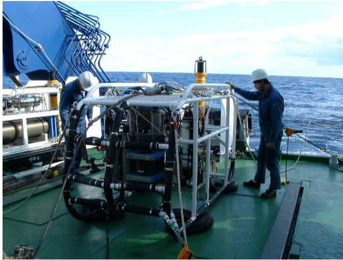
Deep Tow camera ディープ・トウ カメラ
