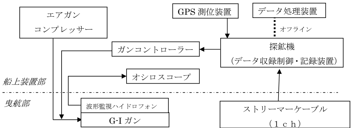
図-4 構成図
