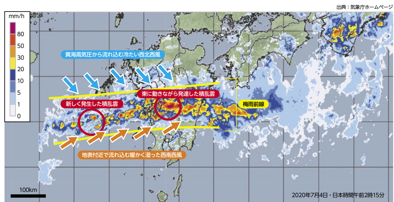
2020年7月、熊本県南部で豪雨が発生していた際の気象庁レーダーによる降水強度分布
