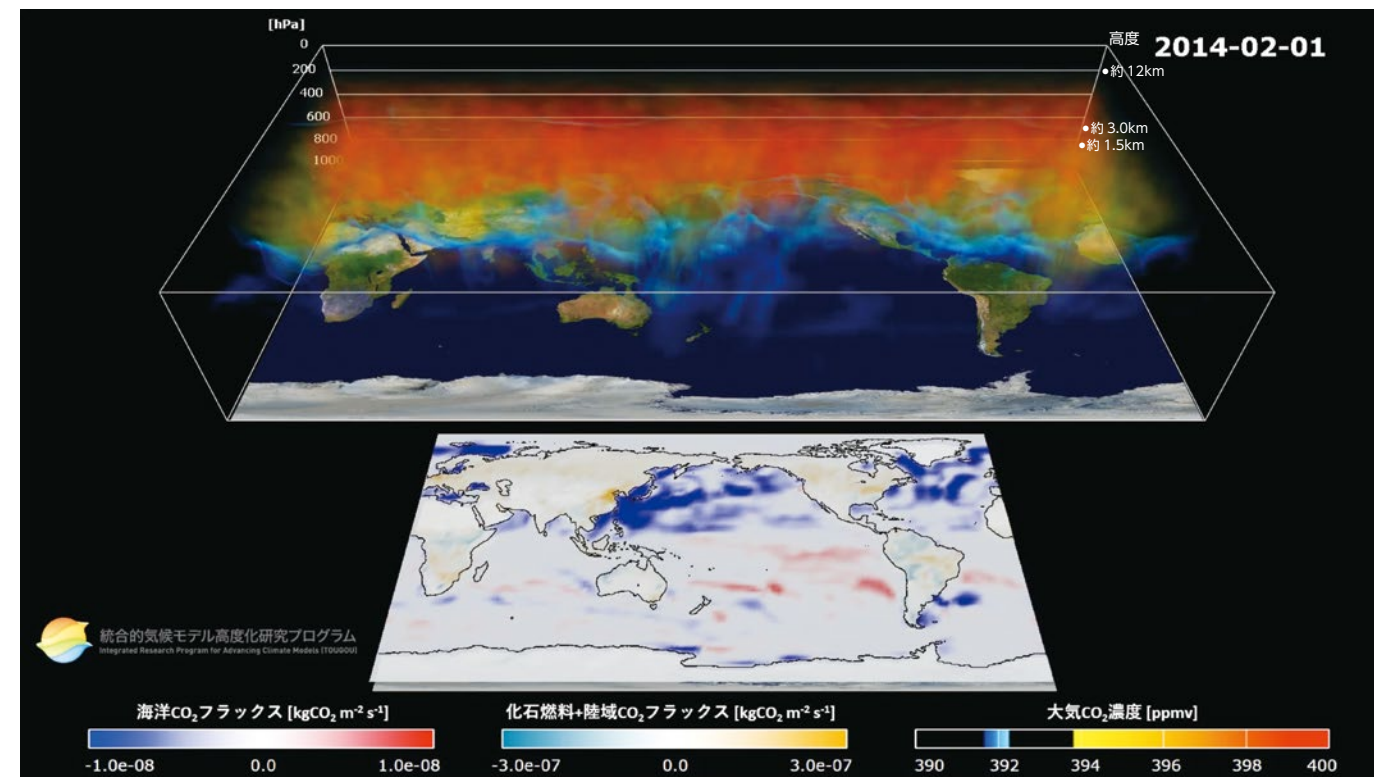
地球システムモデル「MIROC6-ESM」による大気中のCO 2 濃度分布の推定
