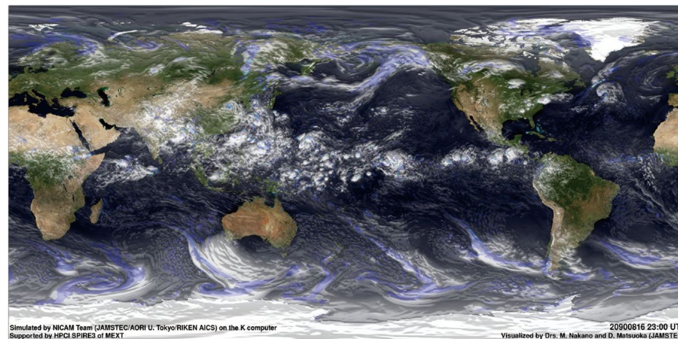
全球雲解像モデル「NICAM」が描き出した地球全体の雲（解像度14km）
