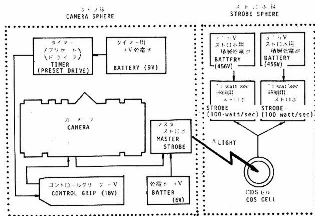
図1 耐圧ガラス球入り深海カメラシステム Deep sea timer drive camera system'
