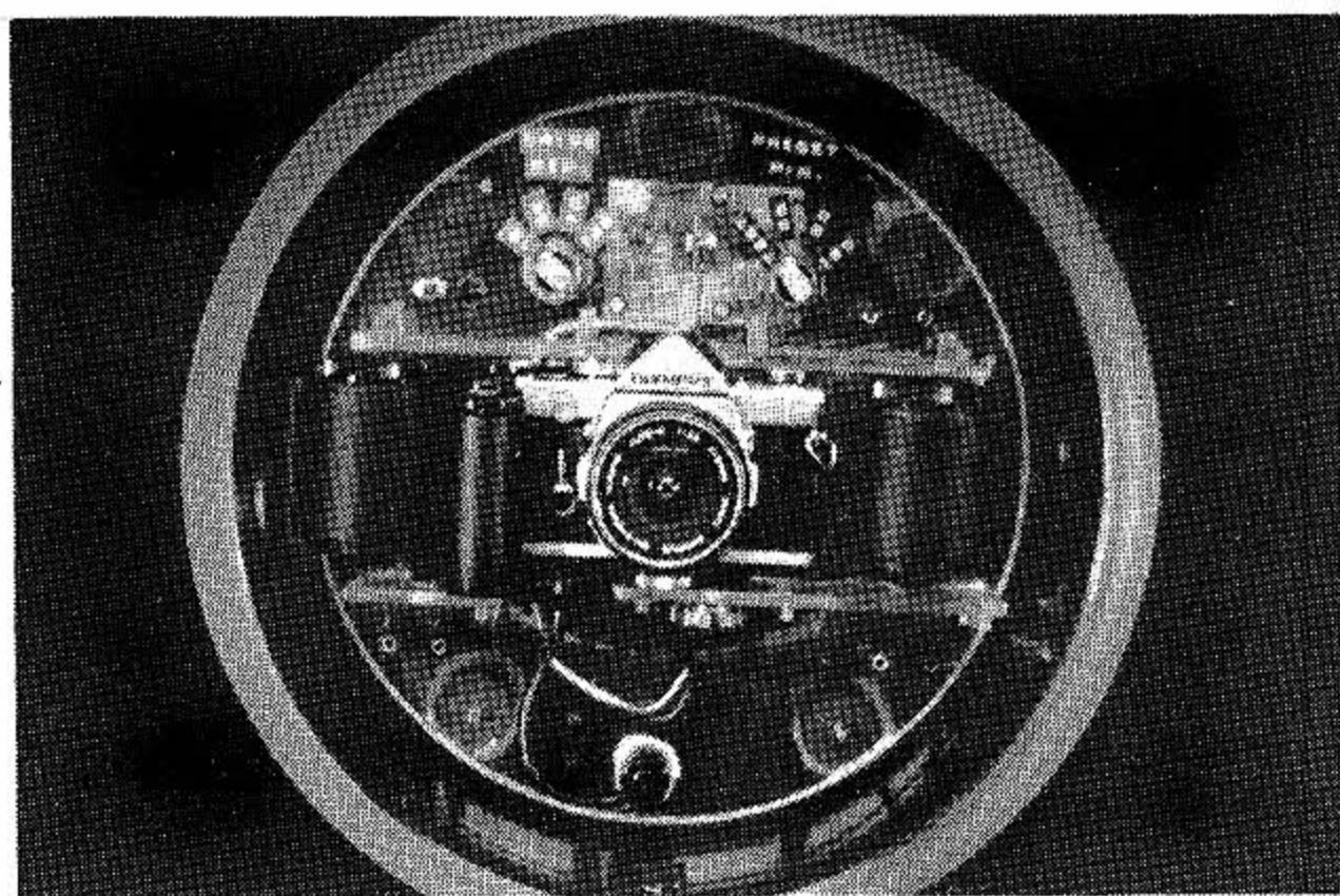
図3 ガラス球にカメラを固定した状態 The Camera in the glass sphere.
