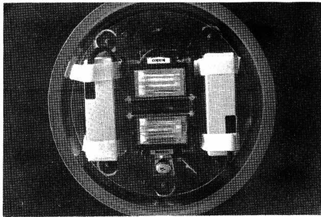
図4 ガラス球にストロボを固定した状態 The strobes in the glass sphere.
