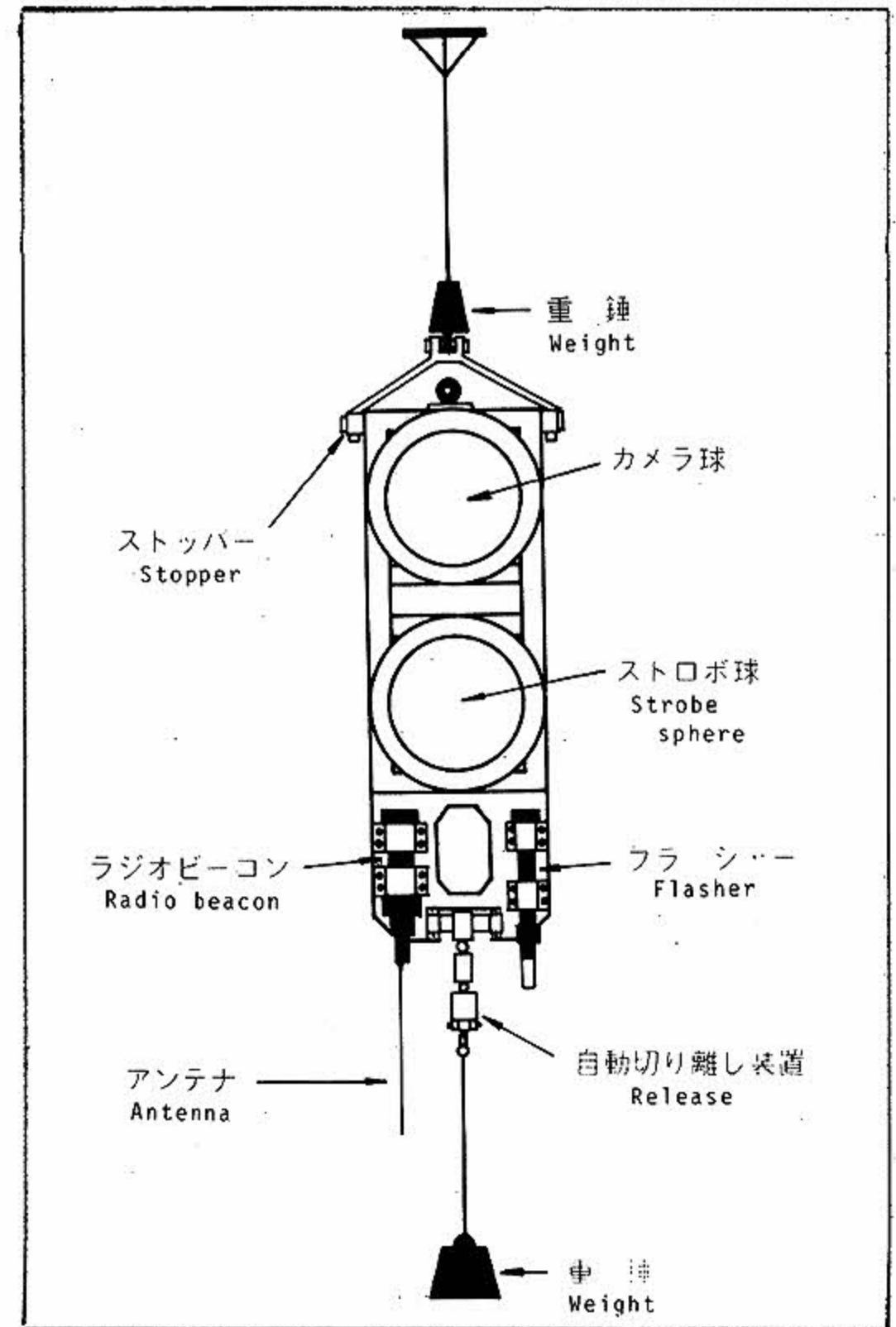
図7 フリーカメラシステム
