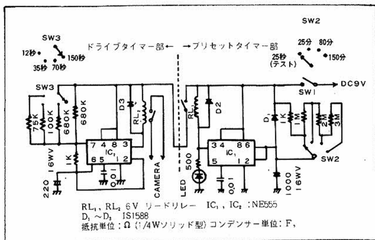
図1 耐圧ガラス球入り深海カメラシステム Deep sea timer drive camera system'
