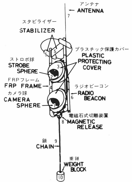
図 3 フリーフォール方式小形耐圧ガラス球入り深海カメラシステム
