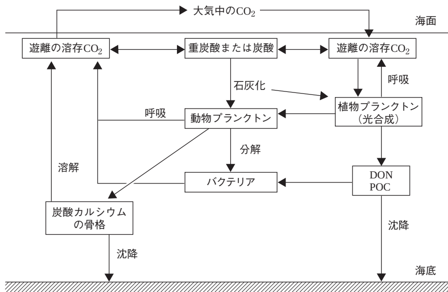
図2.3 海洋生態系における炭素循環 Fig. 2.3 Carbon cycling on the marine ecosystem.
