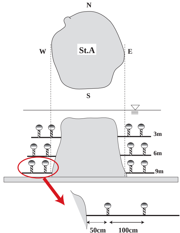
図2 パッチリーフにおける石膏球の設置概略図
