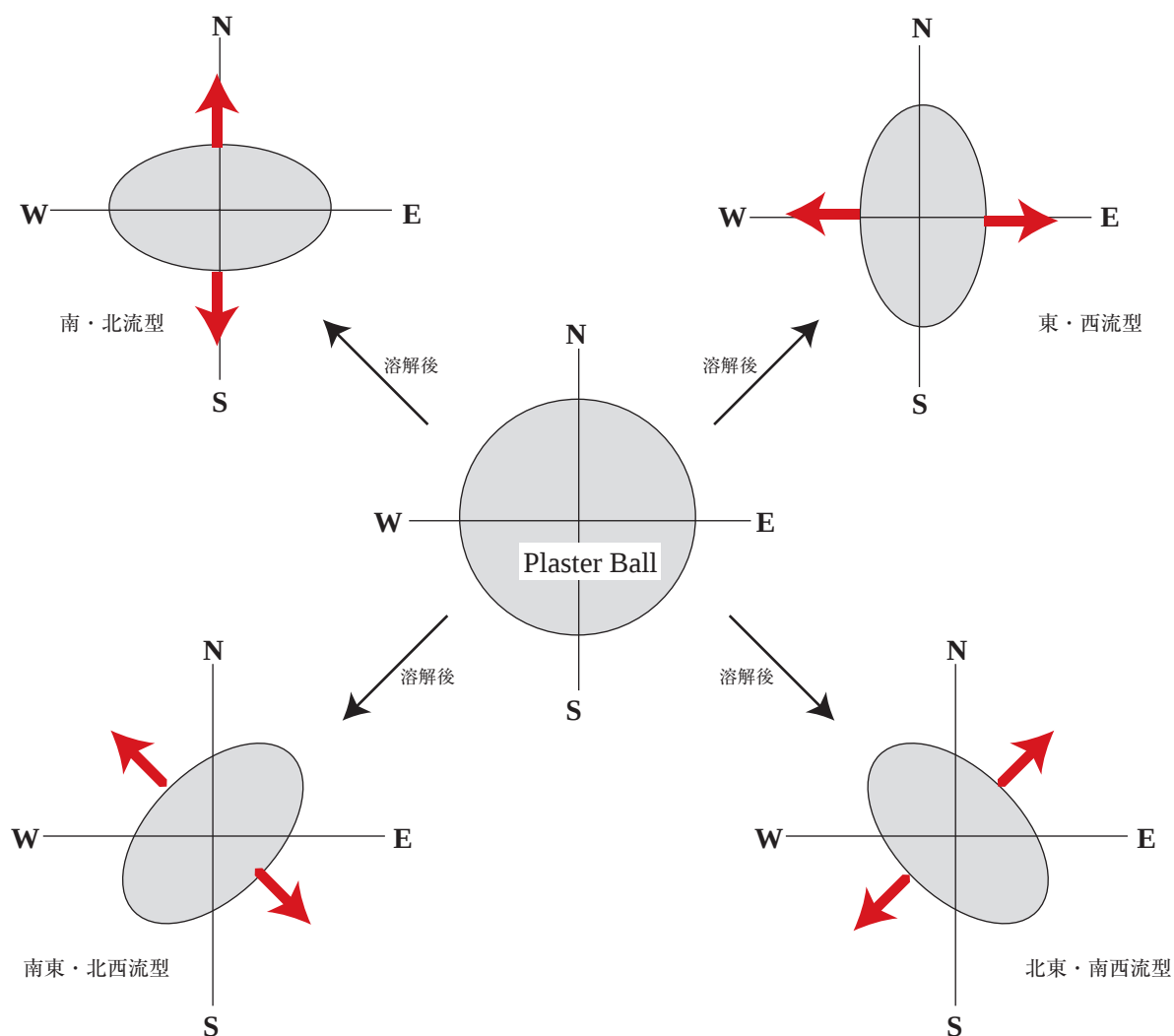
図3 石膏球による流向の決め方の代表パターン
