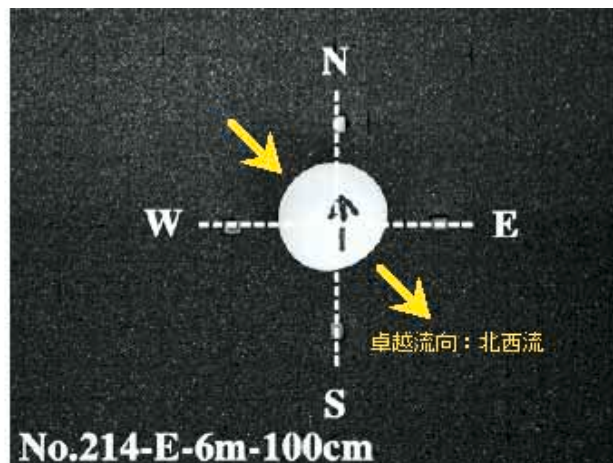
写真2 計測後の石膏球から卓越流向を求める方法の一例
