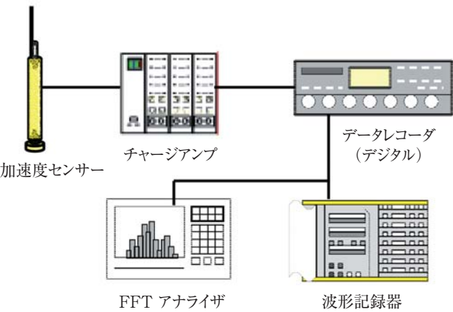
図5 計測システムのブロック図
