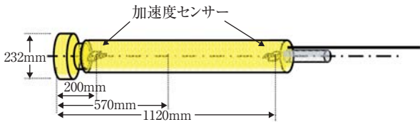
図4c 模擬フロート内部の加速度センサー取り付け位置
