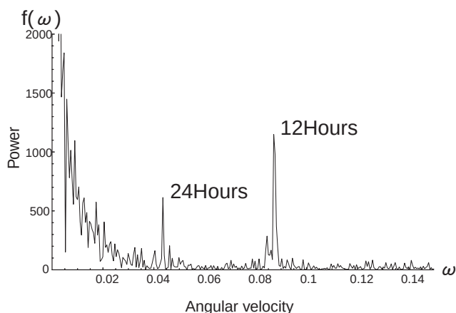
図5 約80日間の水位データから得られたスペクトル分布。
