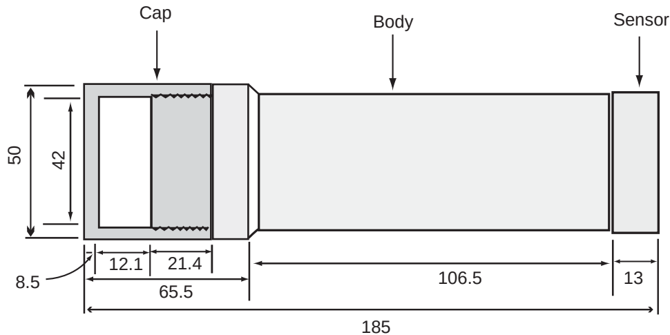
図3 水位計本体(離合社製 RMD-5225A)の構造と寸法 (mm)。
