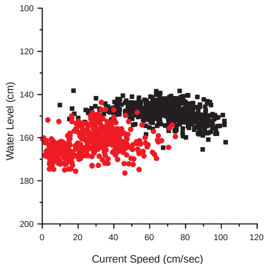
図6 流速と水位データとの関係。■印がはじめの25日間、●印がそれ以降80日までのデータ。
