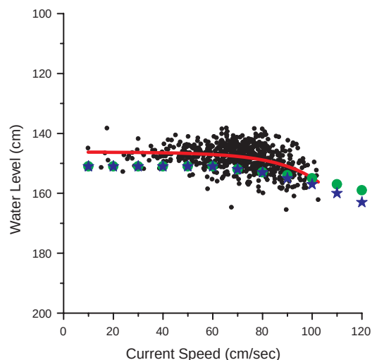
図8 観測された水位と流速との関係(黒点)と指数関数のフィッティング曲線(赤線)。●印は風速を考慮しない場合、★印は風速も考慮した場合の水位のシミュレーション結果。
