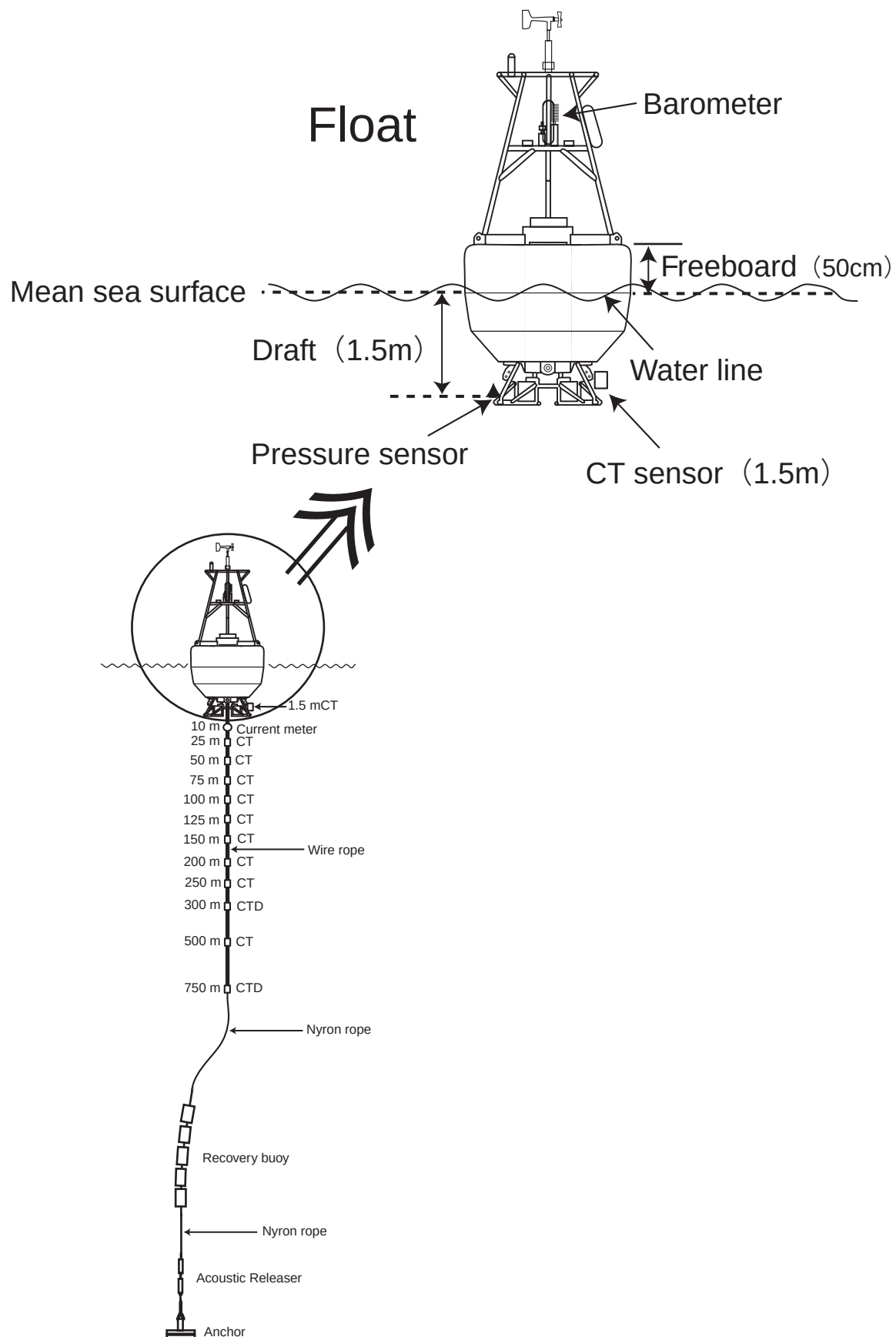
図2 トライトンブイ係留系と今回水位計を取り付けた位置。
