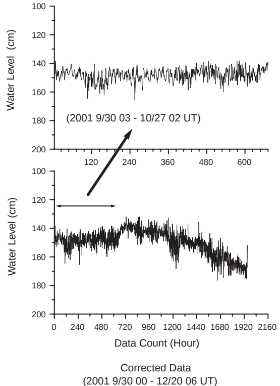
図7 解析に用いた水位データ時系列(上图)。下图は有効な全期間のデータに対して解析に用いたデータの期間(矢印)。
