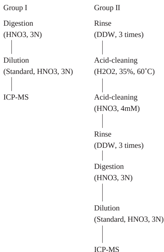
図4 ICP-MS分析試料前処理方法のフローチャート Fig. 4 Flow diagram of chemical procedures for analysis by ICP-MS
