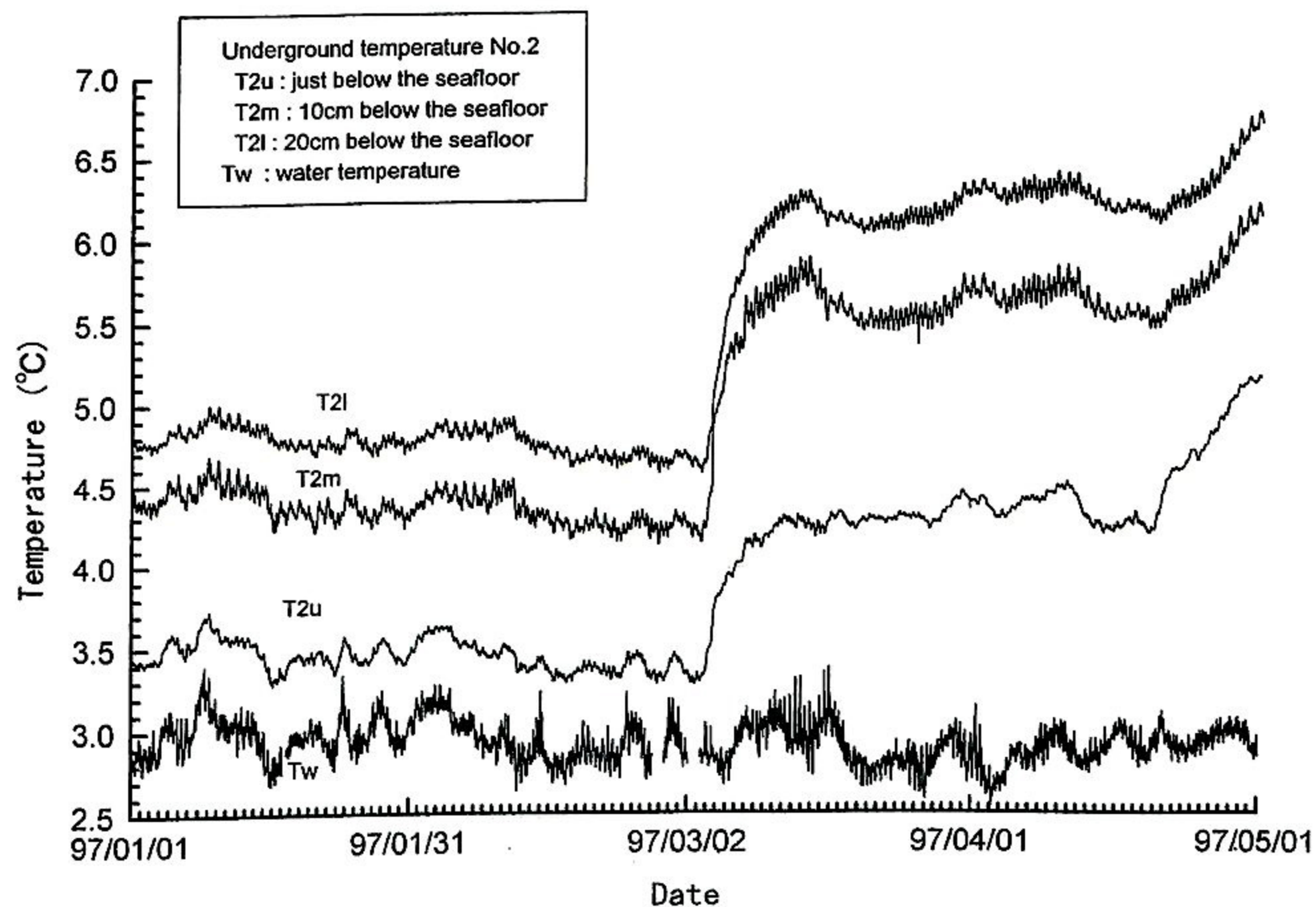
図 7 ステーションによる地中温度計 (No. 2) と水温の記録
