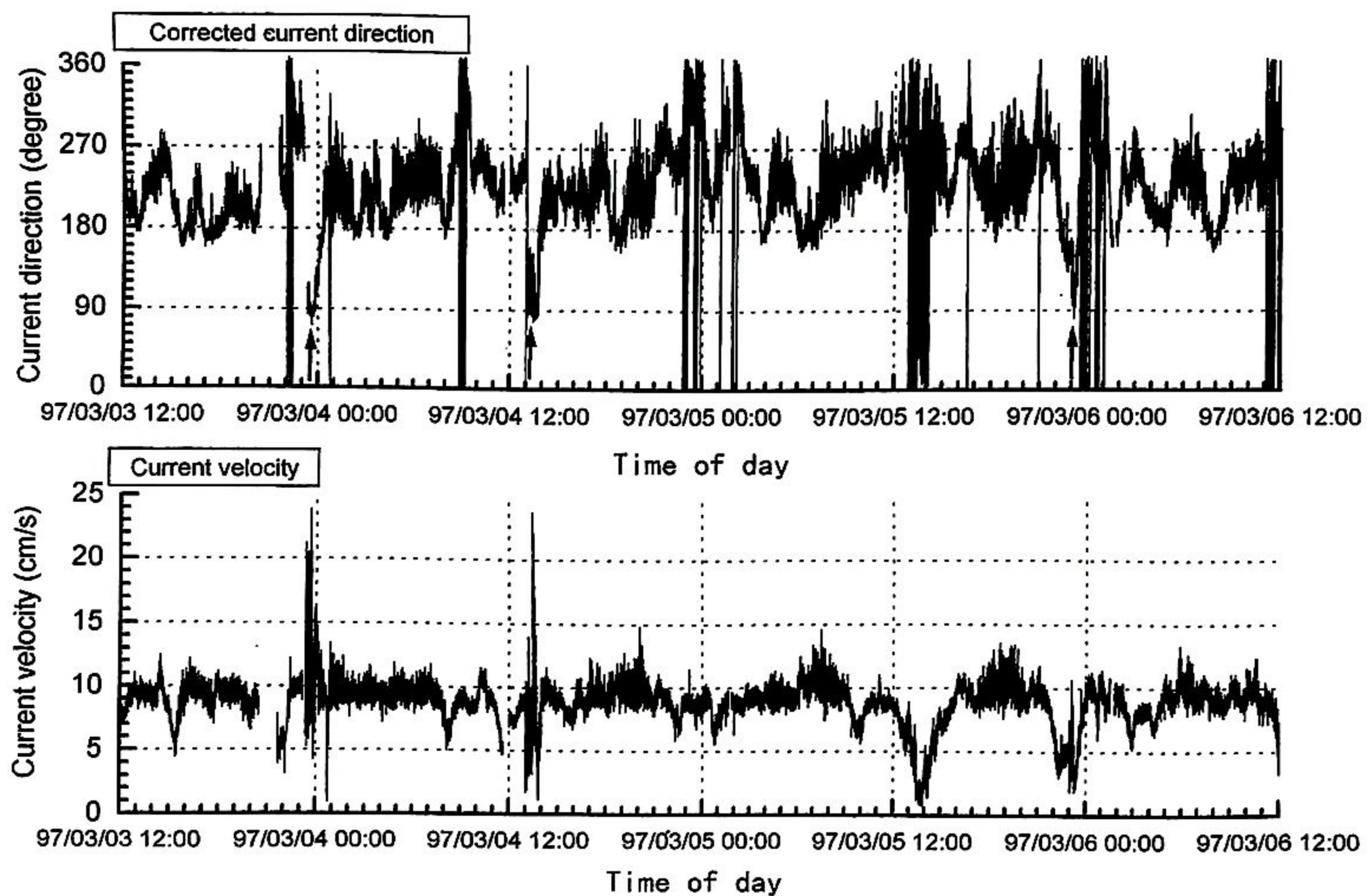
図5 ステーションによる流向・流速記録。矢印は混濁流の発生時を示す
