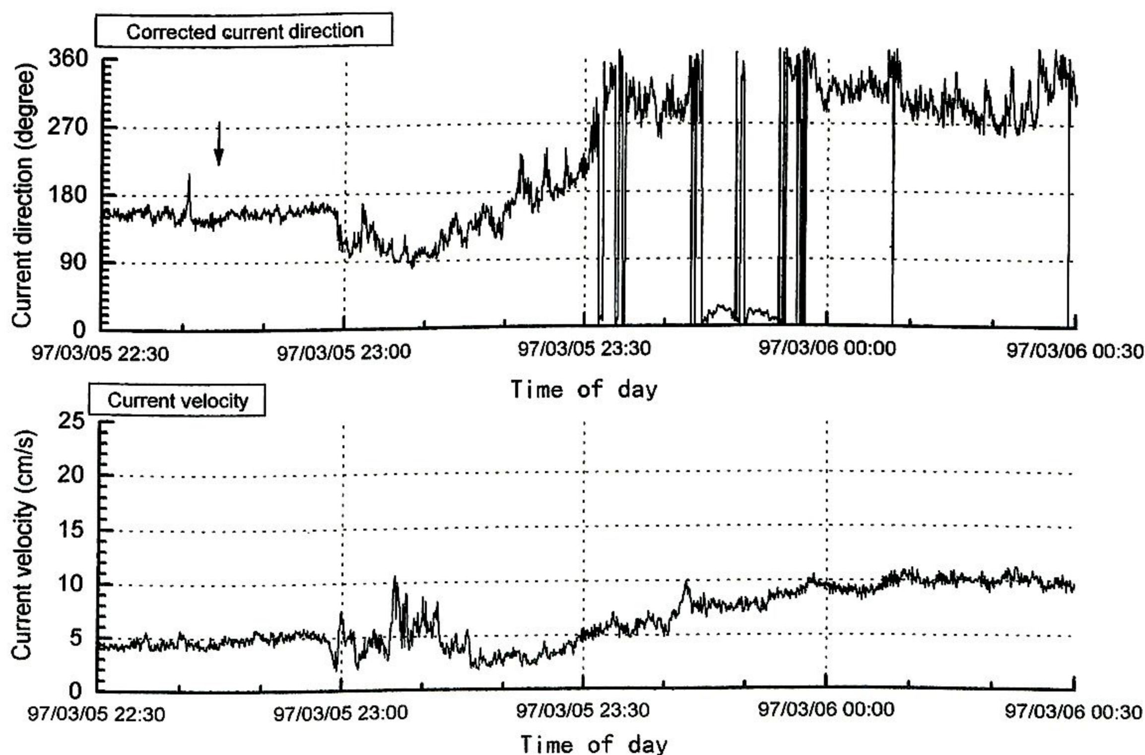
図 4 ステーションによる流向・流速記録。矢印は発震時 (22:43) を示す Fig. 4 Current profile observed by the station. The arrow shows the origin time of the earthquake (22:43).
