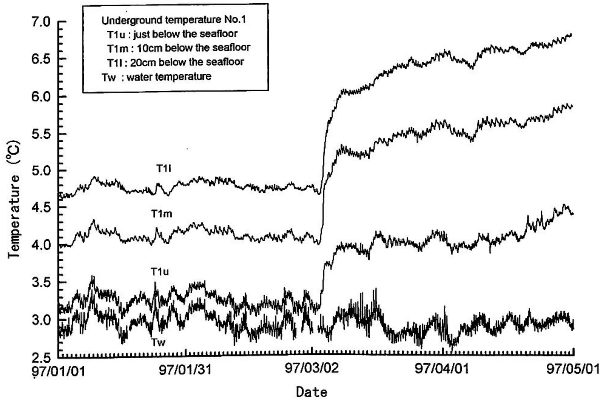
図 6 ステーションによる地中温度計 (No. 1) と水温の記録
