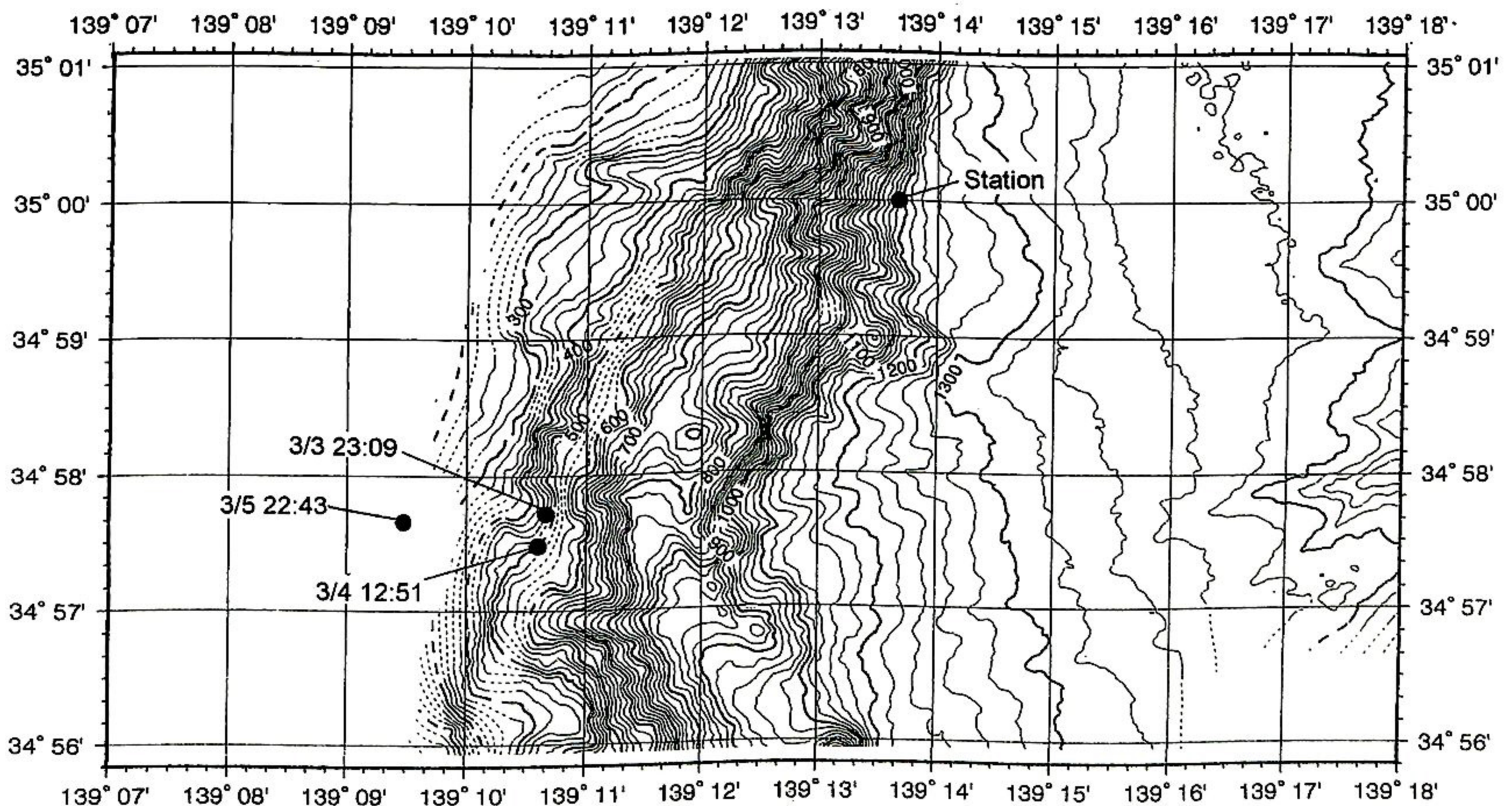
図1 ステーションの位置と混濁流が観測された地震の震央
