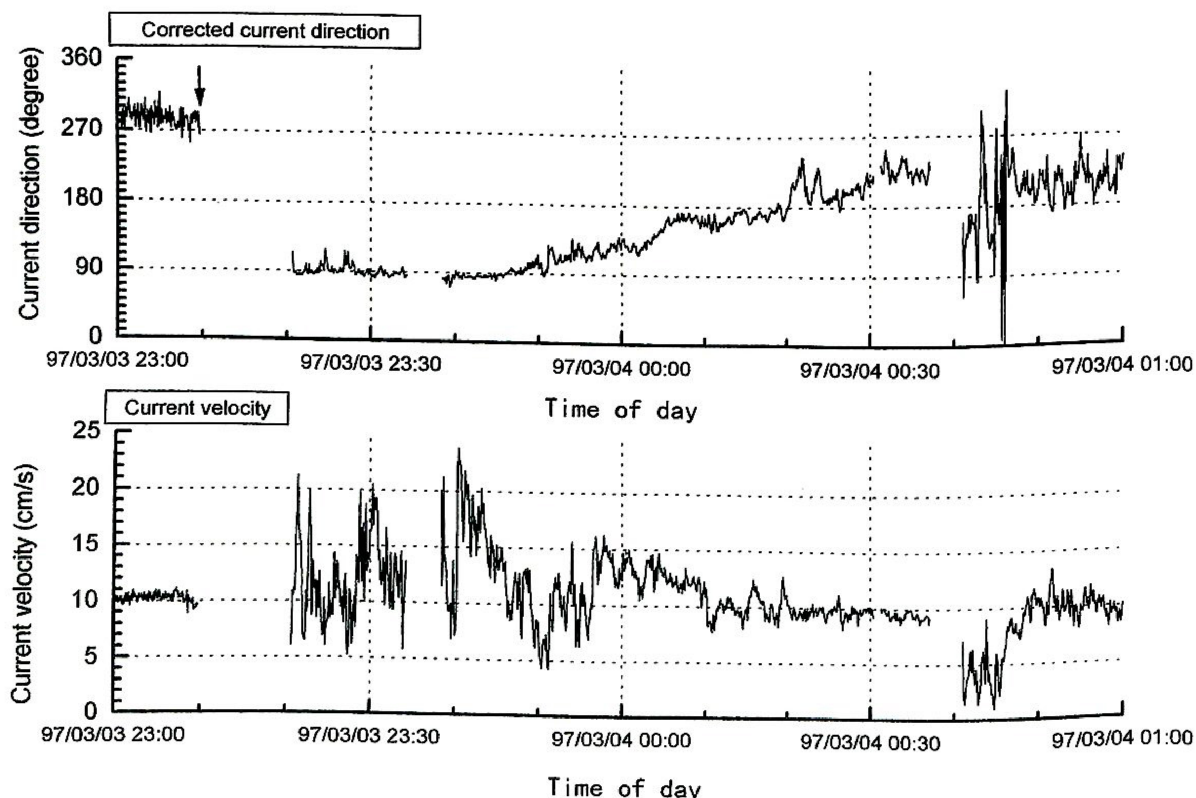
図2 ステーションによる流向・流速記録。矢印は発震時 (23:09) を示す
