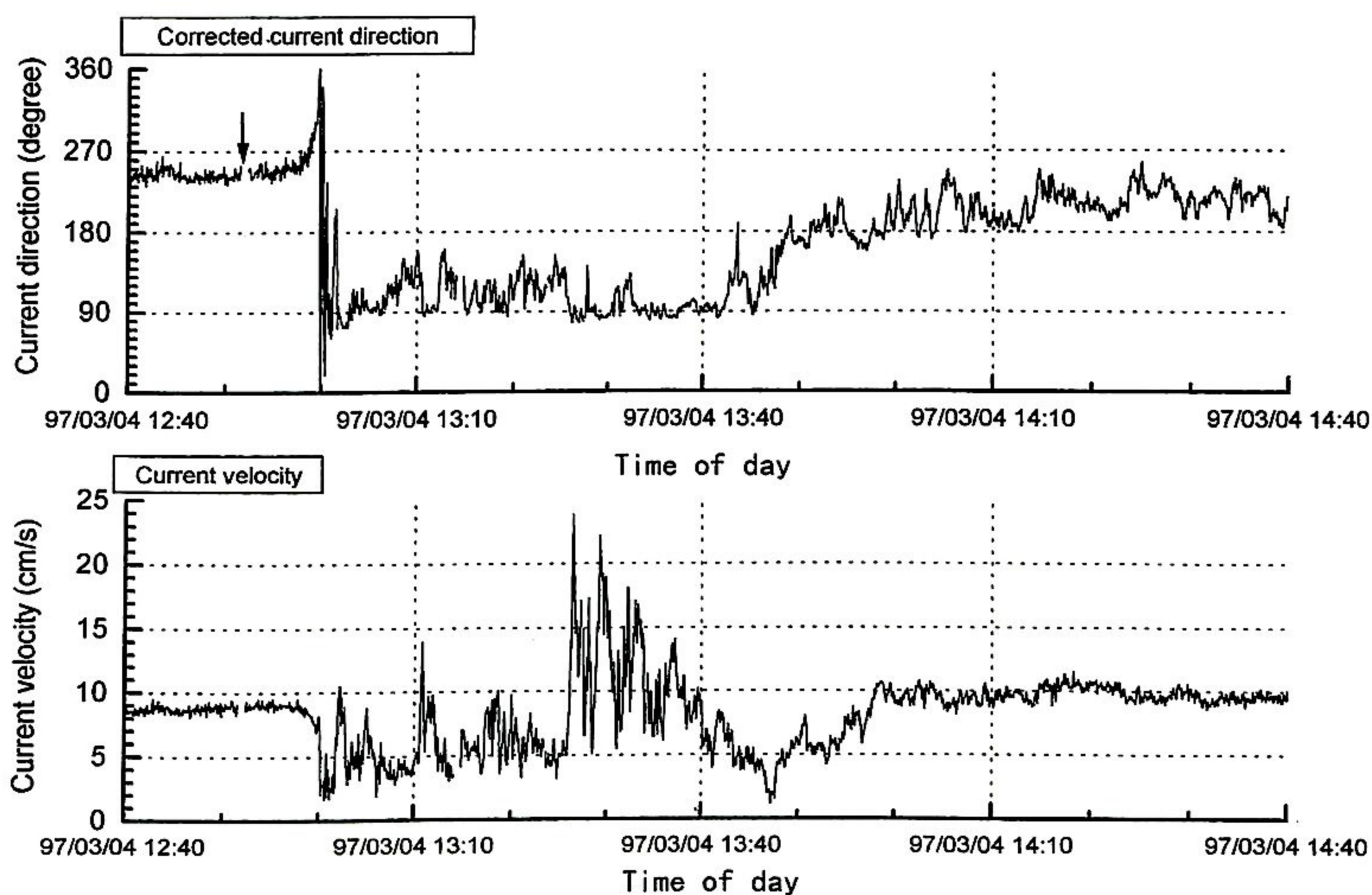
図 3 ステーションによる流向・流速記録。矢印は発震時 (12:51) を示す Fig. 3 Current profile observed by the station. The arrow shows the origin time of the earthquake (12:51).
