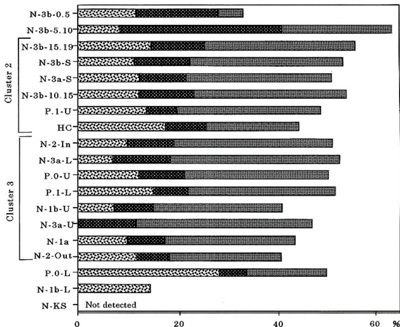
図4 堆積物から抽出した全リン脂質脂肪酸におけるバイオマーカー脂肪酸の割合 (重量%)
