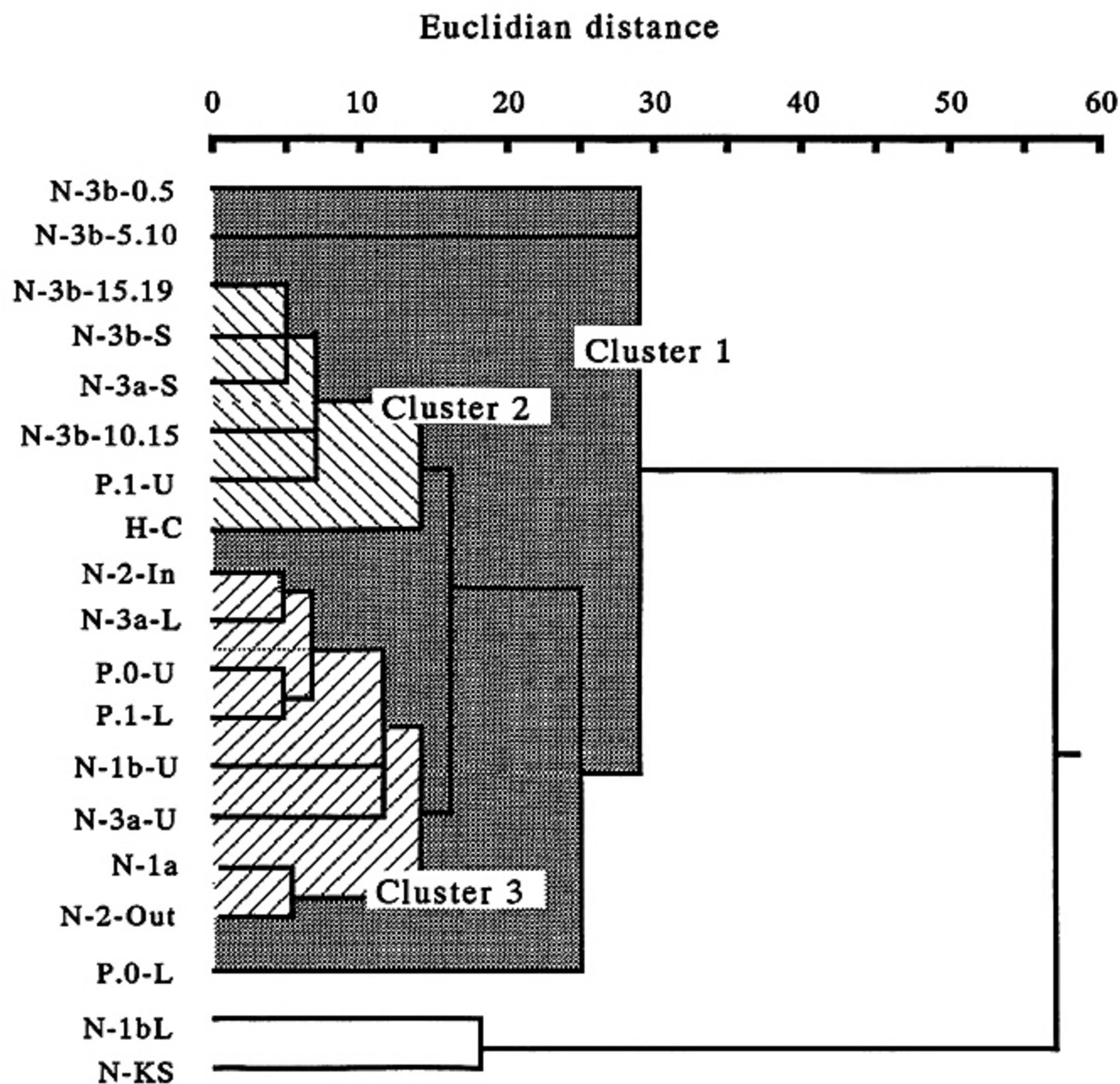
図3 堆積物から抽出したリン脂質脂肪酸の組成にもとづくデンドログラム
