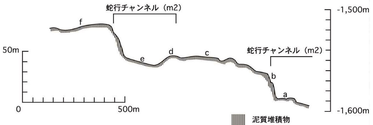
図5 蛇行チャンネル2(m2)での様子。 Fig. 5 submarine surface features (m2).
