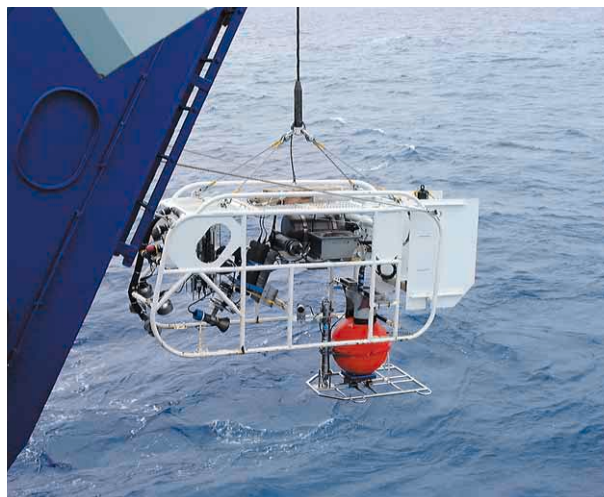
臨時観測装置 (移動部)
