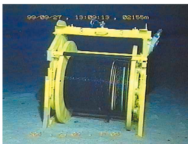
同左（ケーブル展張用ポビン）
