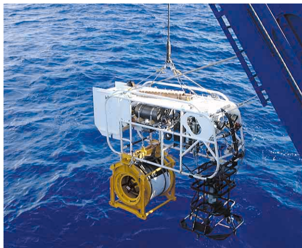
音響測距装置
