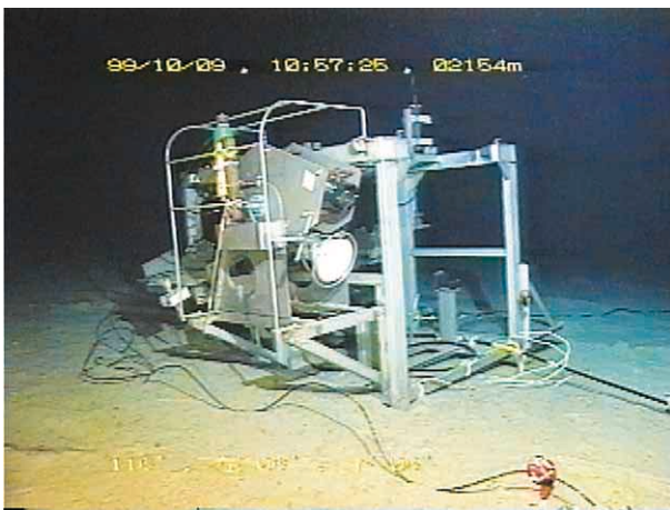
マルチセンサ深海底環境変動観測装置
