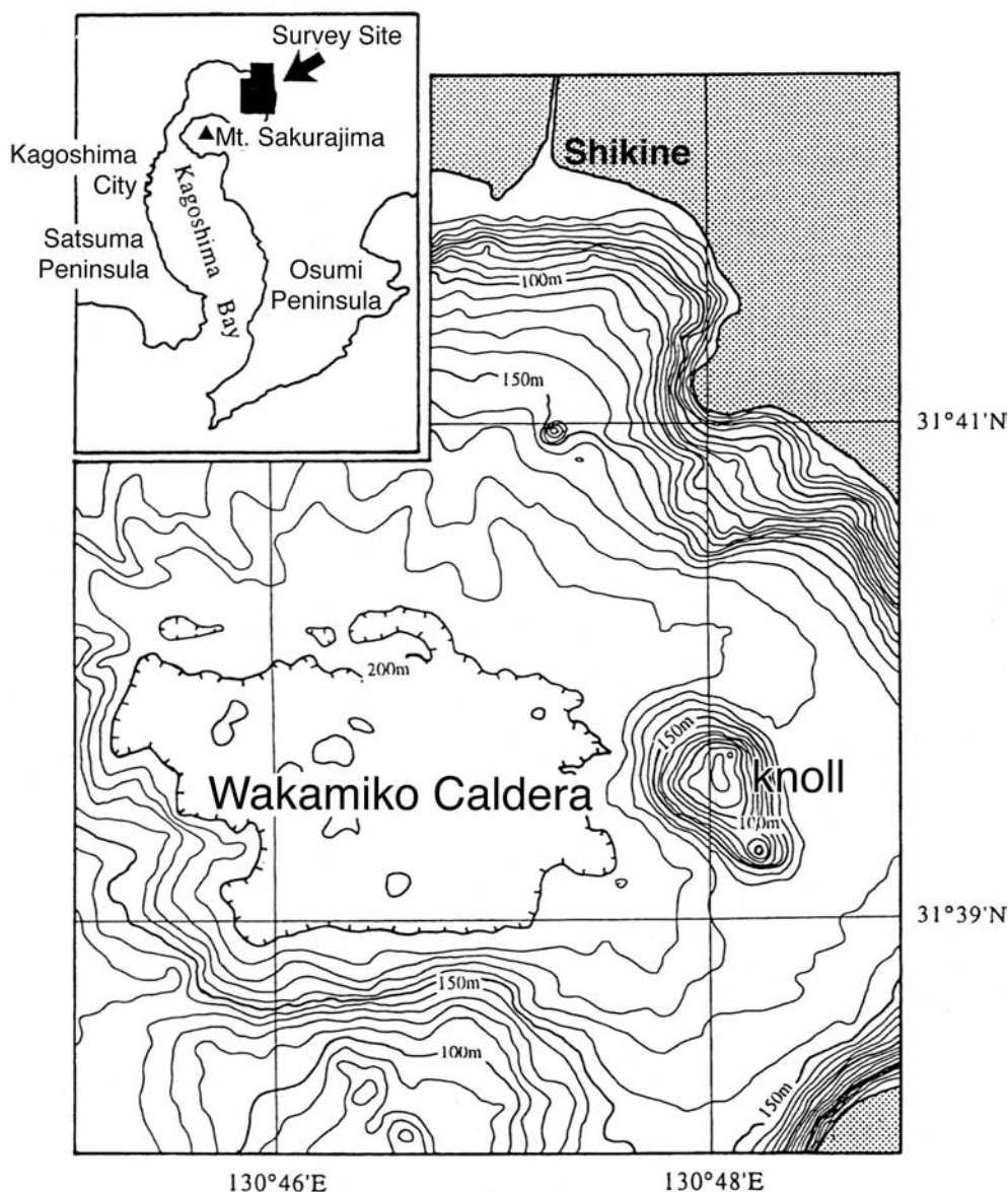
図1 調査海域海底地形
