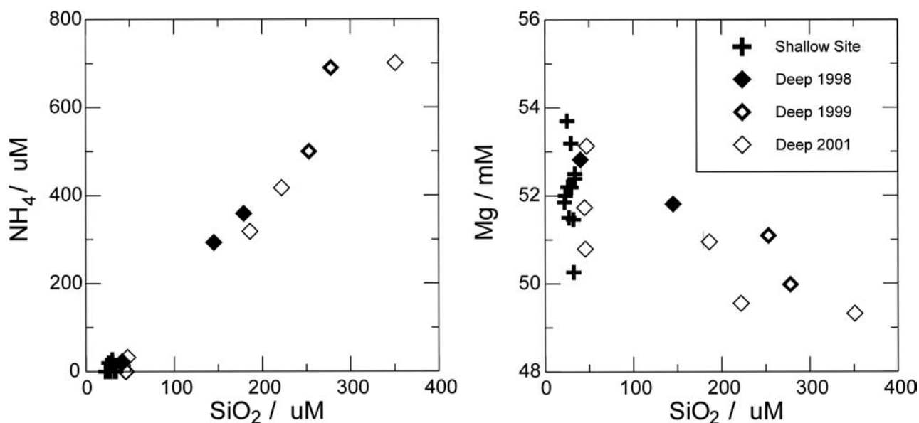
図4 熱水試料の \text{SiO}_2 濃度と \text{NH}_4^+ 濃度との関係(左)およびMg濃度との関係(右)
