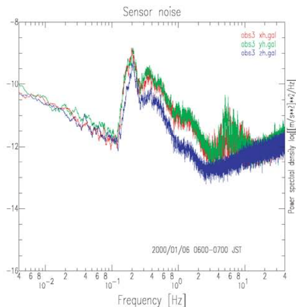
図6 地震計埋設前のOBS3の加速度パワースペクトル密度 Fig. 6 Acceleration power spectrum density of OBS3 before seismometer laying under the seabed.
