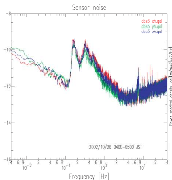
図9 地震計埋設後のOBS3の加速度パワースペクトル密度 Fig. 9 Acceleration power spectrum density of OBS3 after seismometer laying under the seabed.
